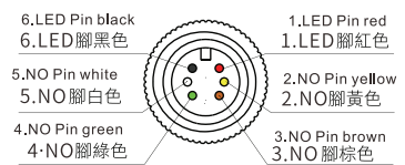
6線單色腳位
