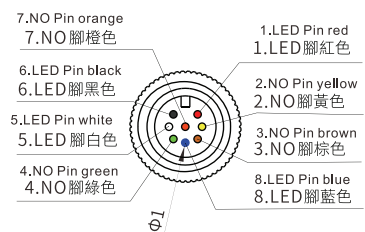
8線三色腳位
